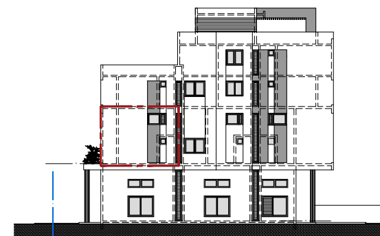
ELEVATION 2
